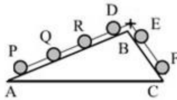
圖 2：史蒂文的斜面規則——兩斜面支撐的重量與所在斜面長度成正比
