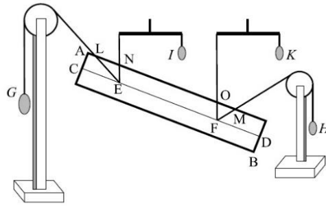
圖 4：由兩傾斜繩子所支撐的平衡柱
